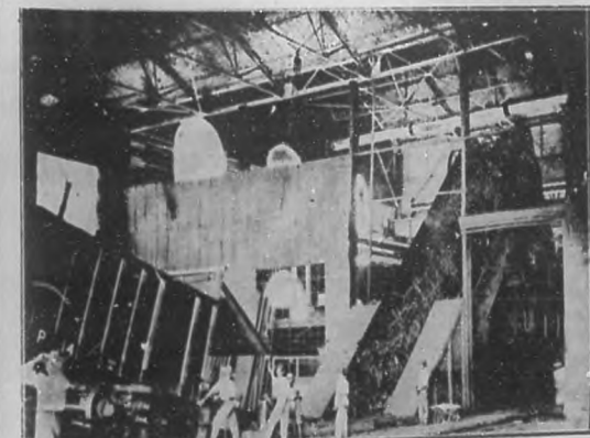
EL CENTRAL "FE".—Trasbordador de caña, del Central "Fe", de la "Sugar Corporation".
