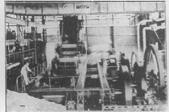
EL CENTRAL "FE".—Vista del nuevo tándem, con tres molinos y dos desmenzadoras, instalado en el gran Central "Fe", de la "Sugar Corporation".
