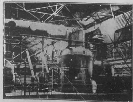
EL CENTRAL "FE".—Vista de los tachos instalados en el Central "Fe", de la Sugar Corporation.
