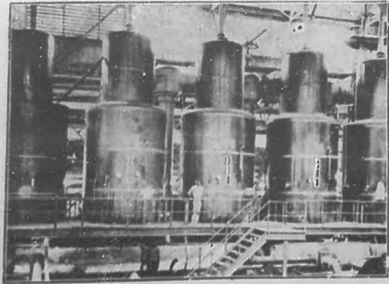
EL CENTRAL "FE".—Una vista de las cuadruple-efecto instaladas en el Central "Fe" de la "Sugar Corporation."
