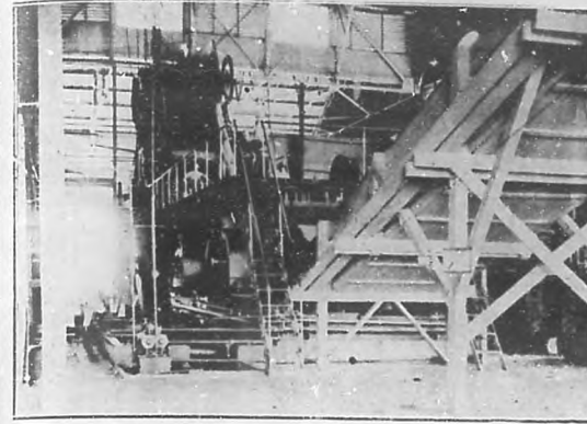
EL CENTRAL "FE".—Otra vista del nuevo tándem instalado en la gran casa de máquinas del Central "Fe".
